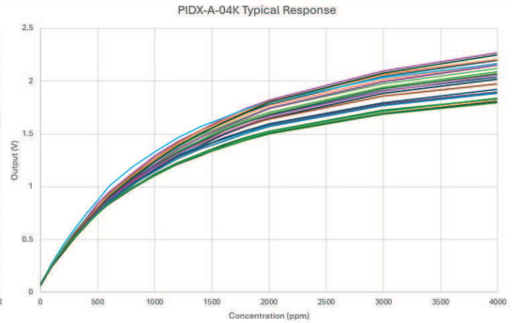
图2 PIDX-A-04K响应 (0-4000 ppm)
