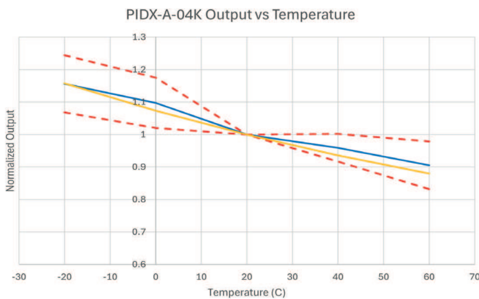
图3 灵敏度温度依赖性
