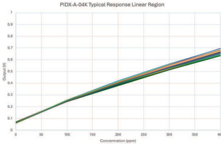
图1 PIDX-A-04K响应 (0-400 ppm)
